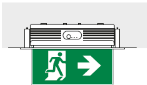
Deckeneinbaumontage Einbaurahmen, weiß Kunststoff Ausschnitt: L 330 x B 70mm Abmessungen Außen: L 360 x B 90
