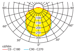
Leuchtmittel: 30W LED-Leiste Deckenmontage
