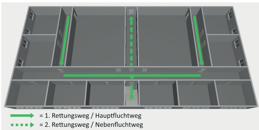
Bild 3.3a: 1. und 2. Rettungsweg / Haupt- und Nebenfluchtweg
