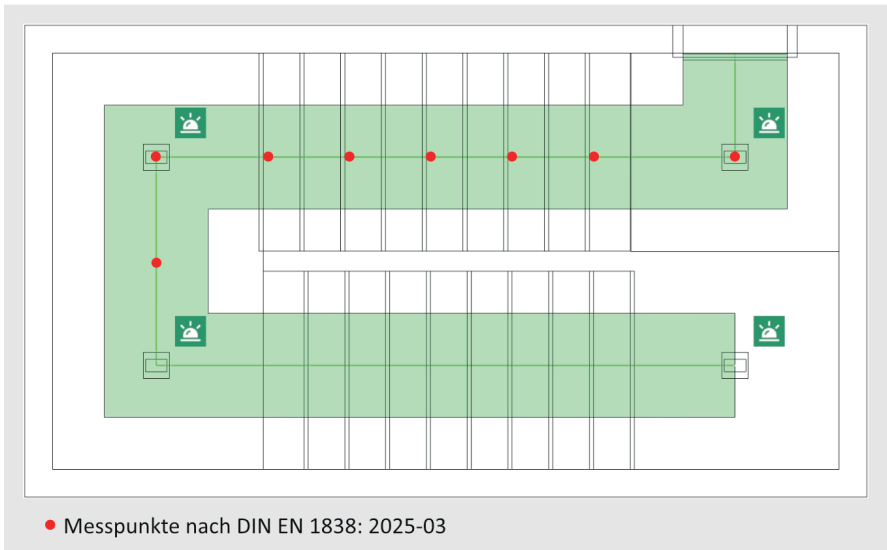
Bild 9.2a: Messpunkte für die Erstmessung in Treppenräumen nach DIN EN 1838: 2025-03
