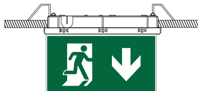
Montage in abgehängter Decke mit Kennzeichnungspanel SP-1100
