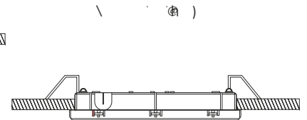
Installation in abgehängter Decke mit Befestigungsfedern A-3018
