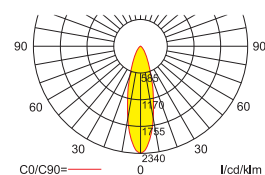
Lampenlichtstrom: 280 lm
