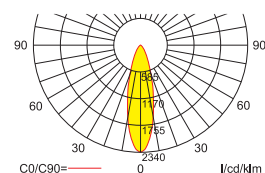
Lampenlichtstrom: 120 lm
