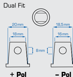
F13 (Schraubanschluss M5)
