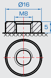
F12 (Schraubanschluss M8)
