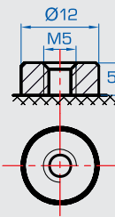
F13 (Schraubanschluss M5)
