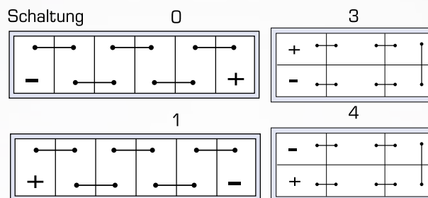
Bodenleiste B1
