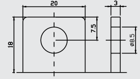
F5 (Anschluss Fahne)
