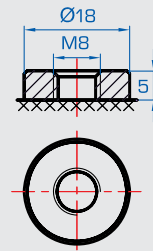
F14 (Schraubanschluss M8)
