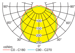
Leuchtmittel: 1,5W LED-Leiste Deckenmontage
