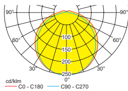
Leuchtmittel: 6W LED-Leiste Deckenmontage
