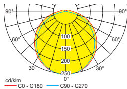
Leuchtmittel: 1,5W LED-Leiste Deckenmontage
